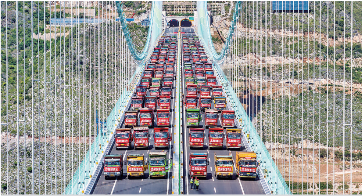
8月25日拍摄的贵州花江峡谷大桥荷载试验现场。8月25日，在建世界第一高桥——贵州花江峡谷大桥荷载试验顺利完成，通车在即。在静力荷载试验过程中，96辆总重达3300吨的重型大货车分批驶上桥面，对大桥进行了一次全面而严格的“体能测验”。荷载试验顺利完成，标志着大桥通过了通车前的“关键大考”，有望于9月下旬宣布通车。花江峡谷大桥于2022年1月开工建设，是贵州六枝至安龙高速公路的控制性工程，全长2890米，主桥跨径1420米，桥面到水面高度625米。花江峡谷大桥建成后，主桥跨径将居山区桥梁跨径世界第一、桥梁高度将居世界第一。
