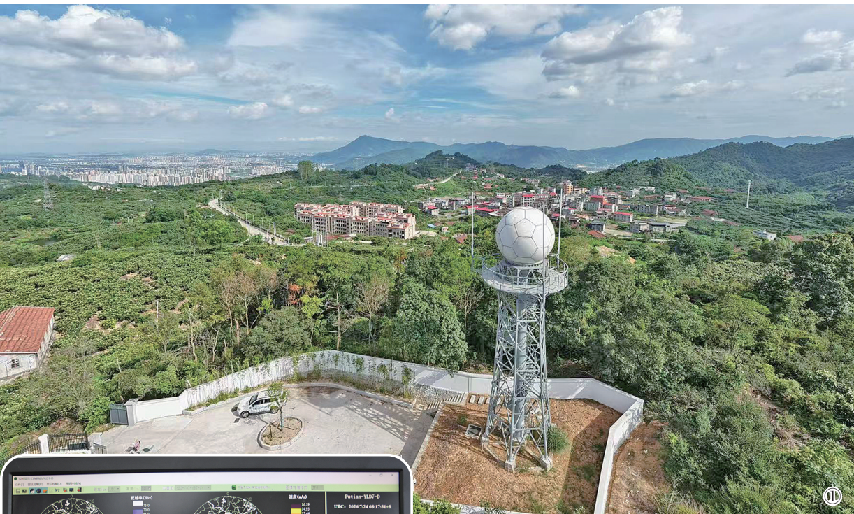
图①:运行的X波段双偏振天气雷达地处海拔400多米的城厢区凤凰山街道白洋村。
